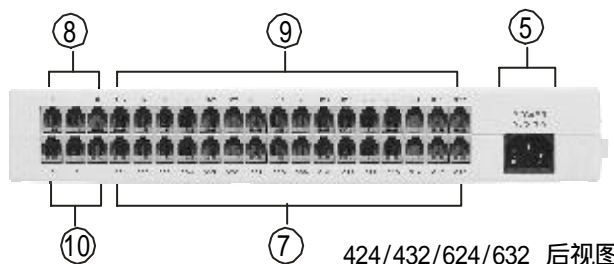
424/432/624/632 后视图
